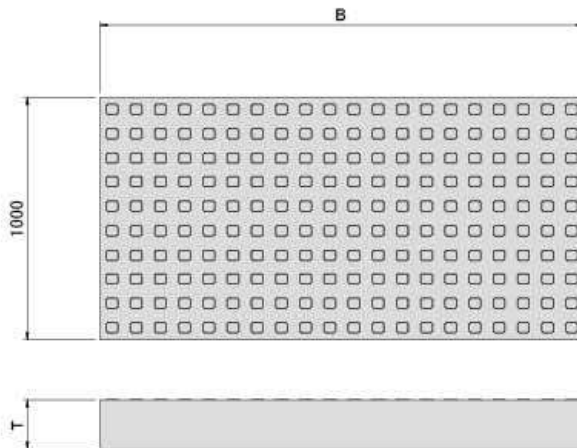
単体図
