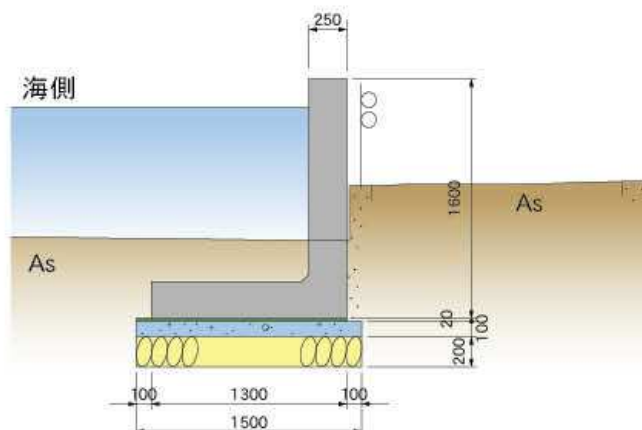
防潮堤
