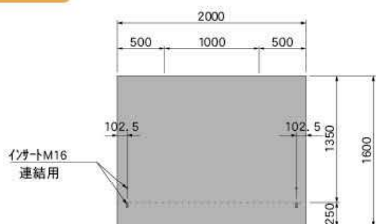
単体図
