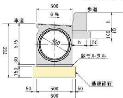
〈VRP-402〉本体標準断面図
