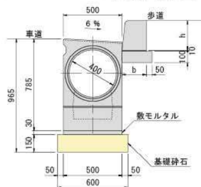
〈VRPG-40〉柵標準断面図
