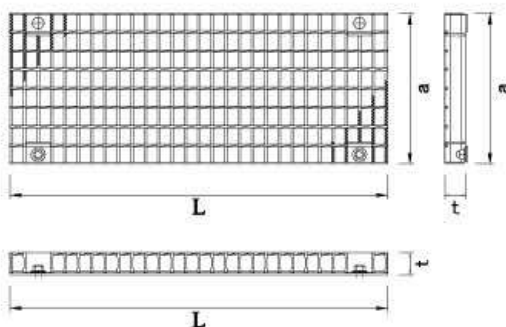
グレーチング (T-25) ボルト固定
