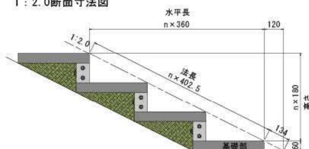
1 : 2.0断面寸法図
