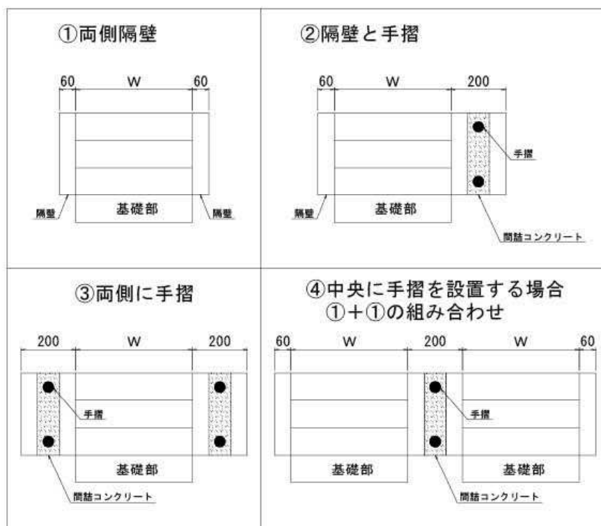
1 : 1.5断面寸法図
