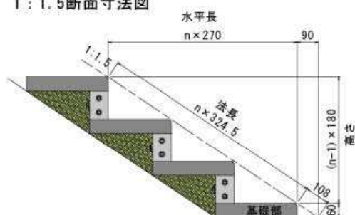
1 : 1.5断面寸法図
