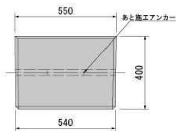
正面図
