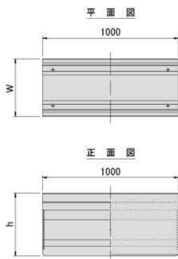
OSU側溝 横断用
