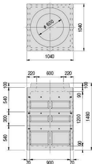
900 × 1200 組み合わせ例図
