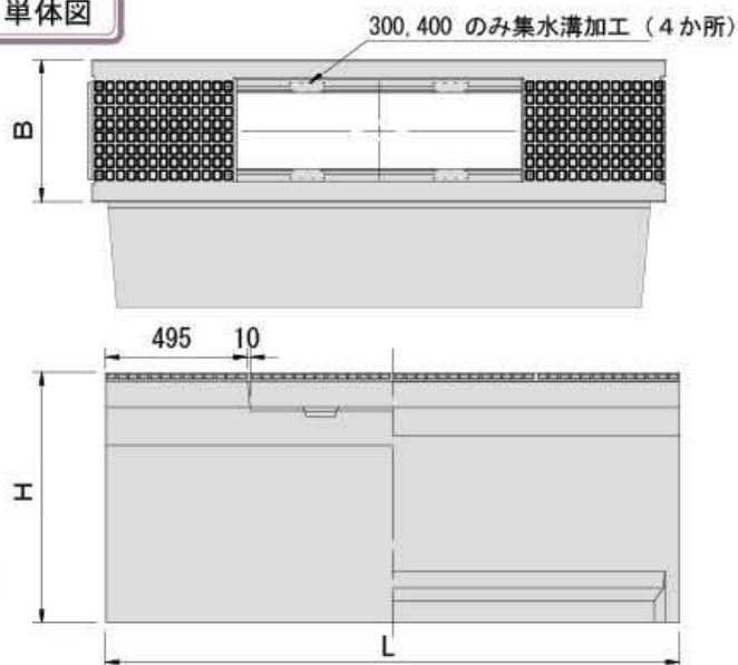
単体図
