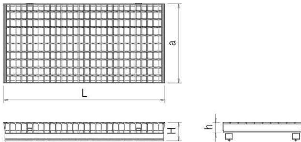
単体図
