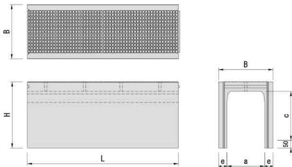
単体図
