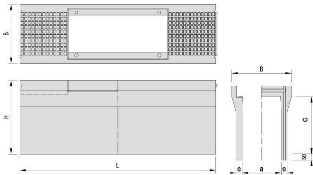
単体図
