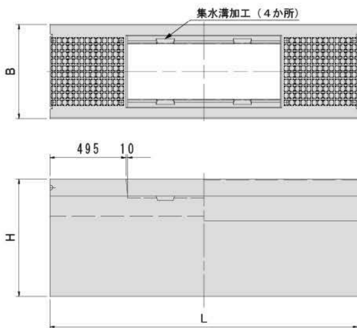
単体図
