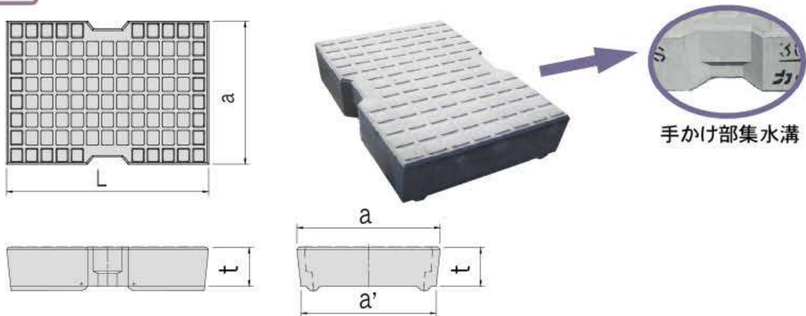
単体図
