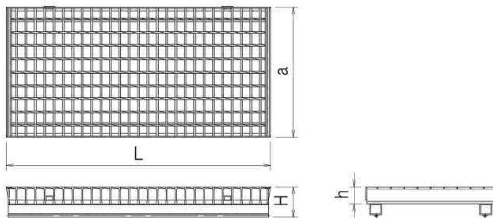
単体図
