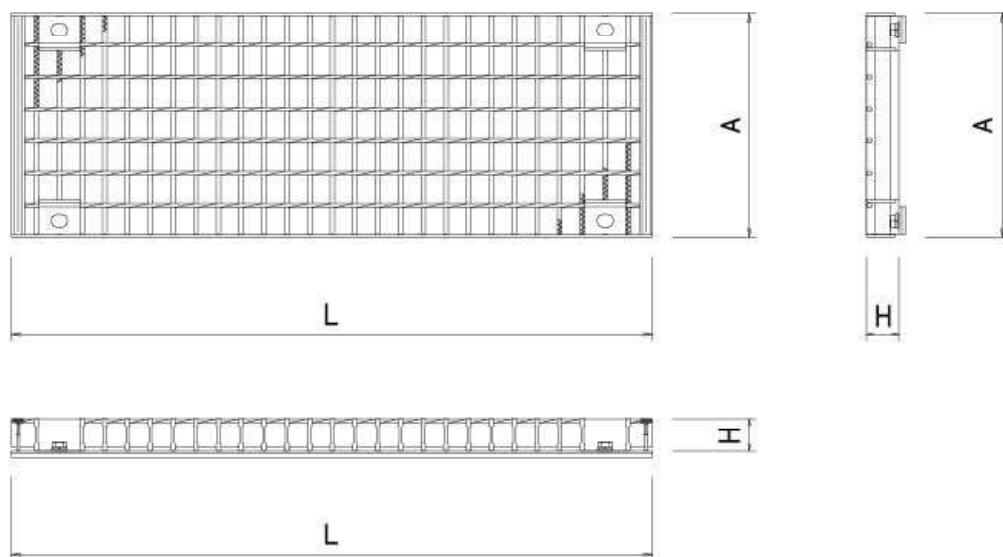
単体図
