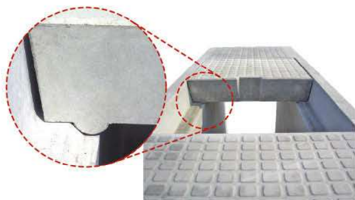
設置状態
